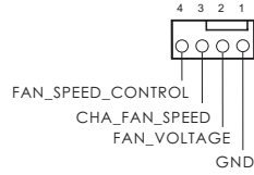
CHA_FAN1
