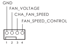
CHA_FAN2
